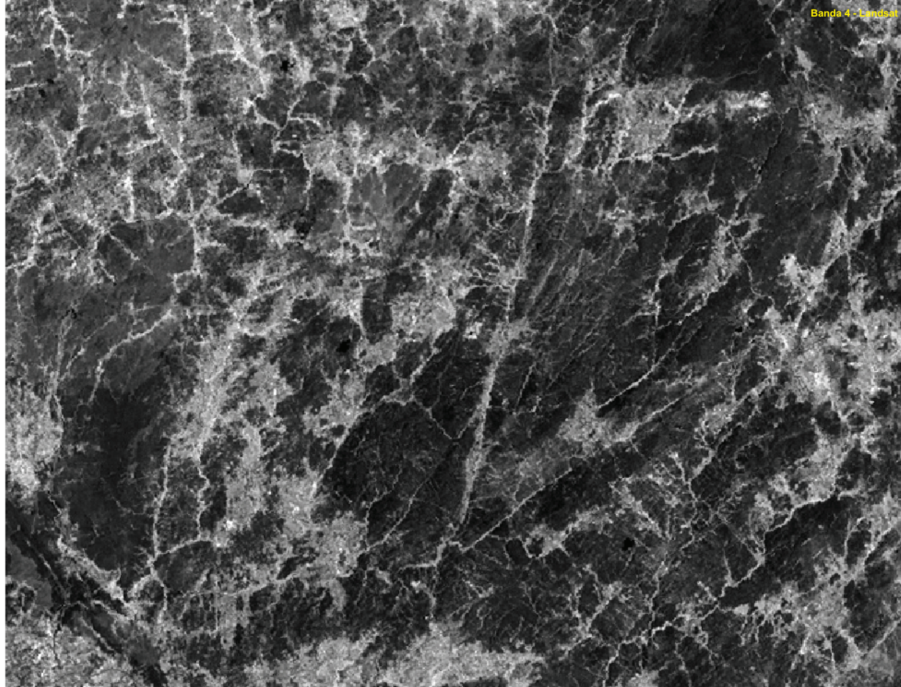
Banda 4 - Landsat
