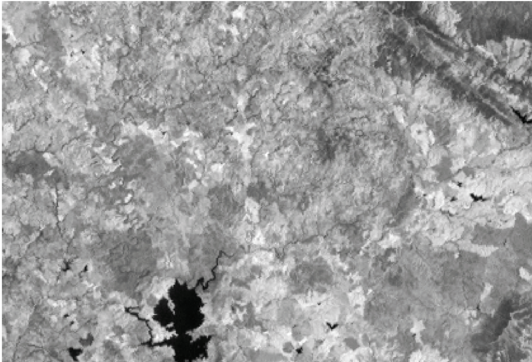
Banda 6-2 - Landsat - contraste linear
